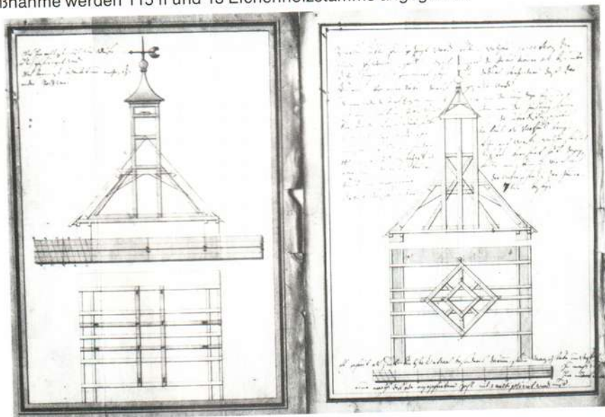
Die beiden Turm-Erneuerungspläne 1790 von Werkmeister Rebstock (rechts) und Landbaubeister Meerwein (links).
